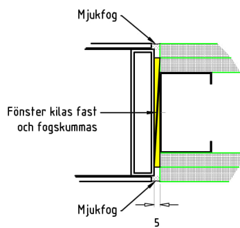
Exempel på anslutning mot platsbyggd gipsvägg
